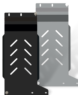
RANGER - FO08.2171 - převodovka (ocel) FO08.2172 - převodovka (AL)
